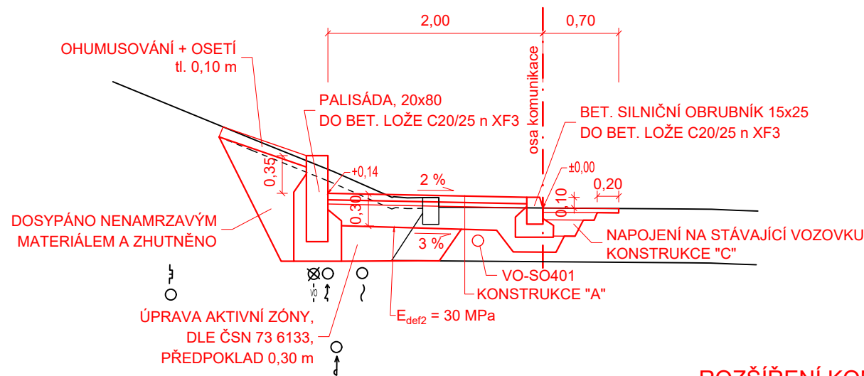
CHODNÍK V ZÁŘEZU km 0,018 20 - km 0,037 20
