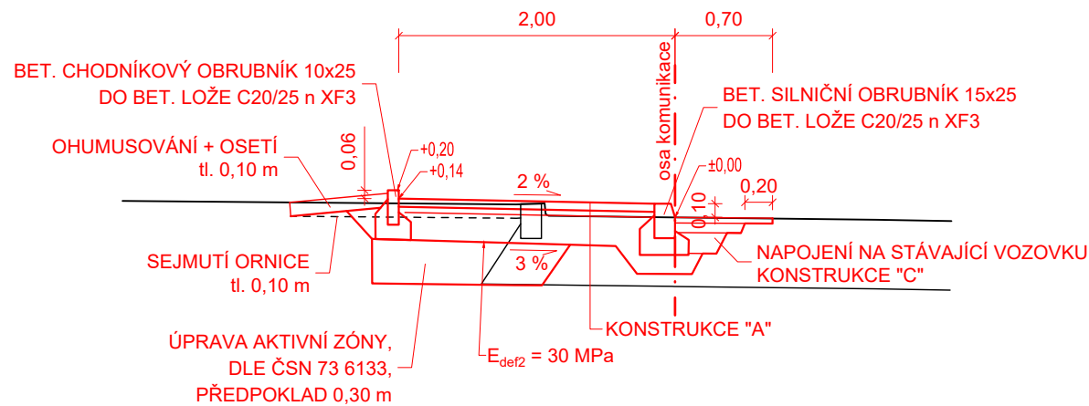
CHODNÍK V ZÁKLADNÍM PROVEDENÍ
