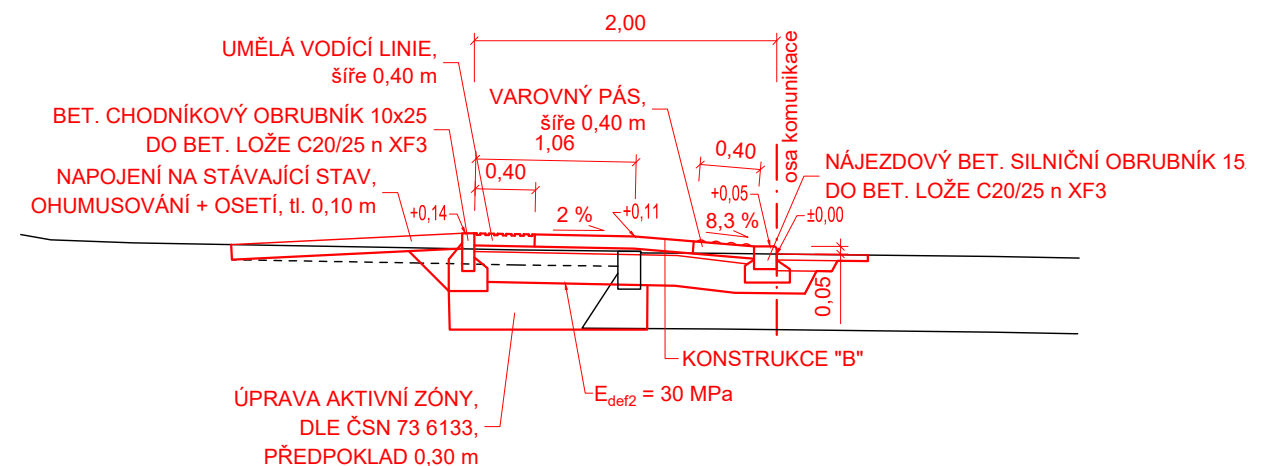
CHODNÍKOVÝ PŘEJEZD samostatný sjezd km 0,042 92
