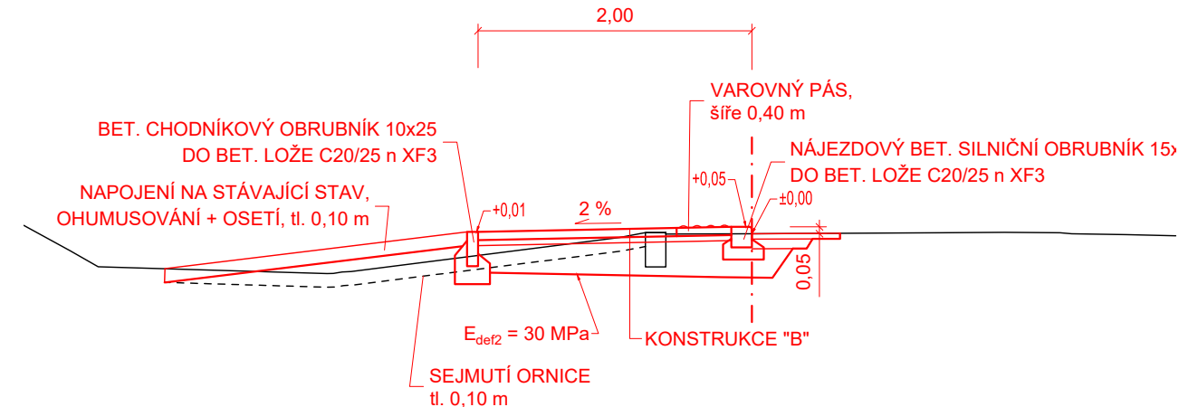
CHODNÍKOVÝ PŘEJEZD samostatný sjezd km 0,064 36
